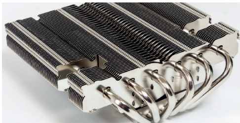
Poput zrcala: Niklom presvučena bakrena baza hladnjaka "zglancana" je skoro do savršenstva
