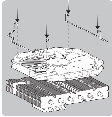
Insert fan clips onto holes of fan
